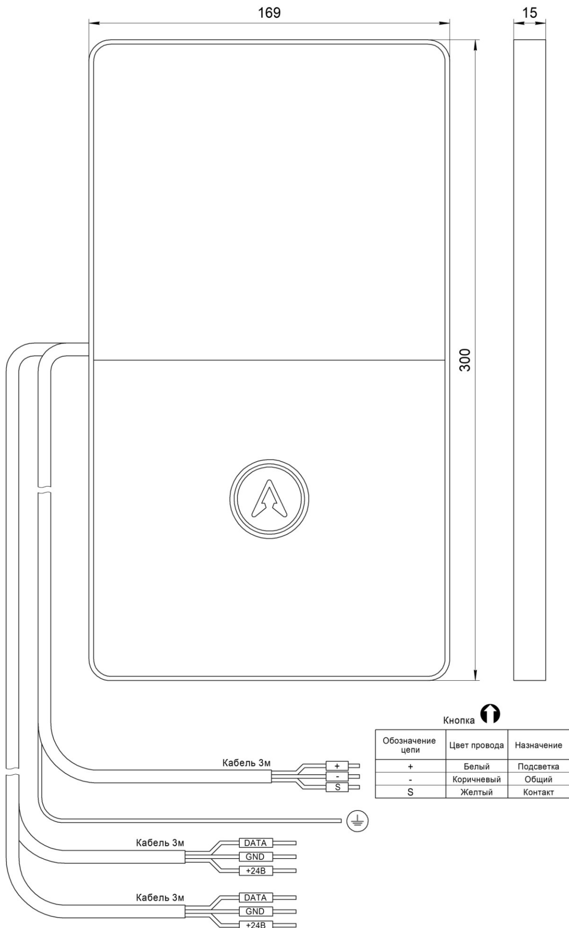
Рис.1 Внешний вид Вызывной пост ОНИКС НШЕК.468381.065
